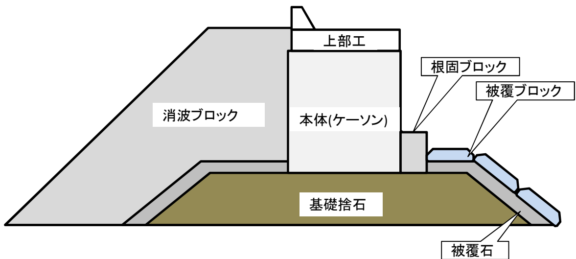
防波堤(混成堤)一般構造図
